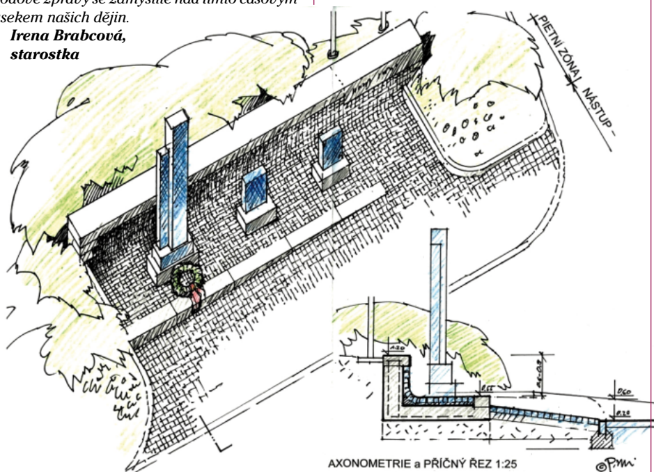
AXONOMETRIE a PÍČNÝ REZ 1:25
